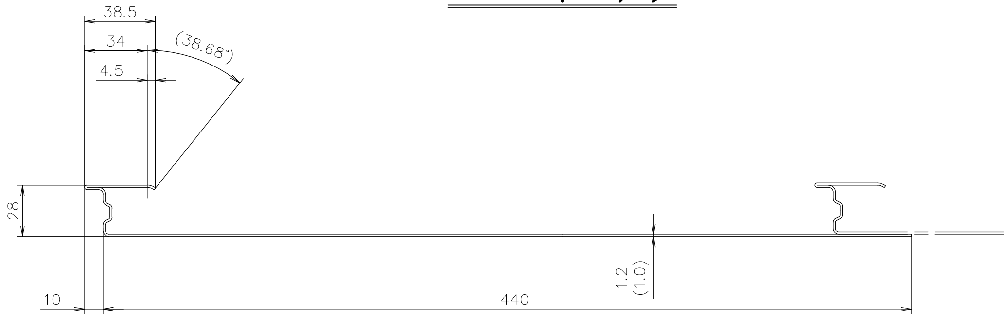
全 景 図 (S=1/6)
