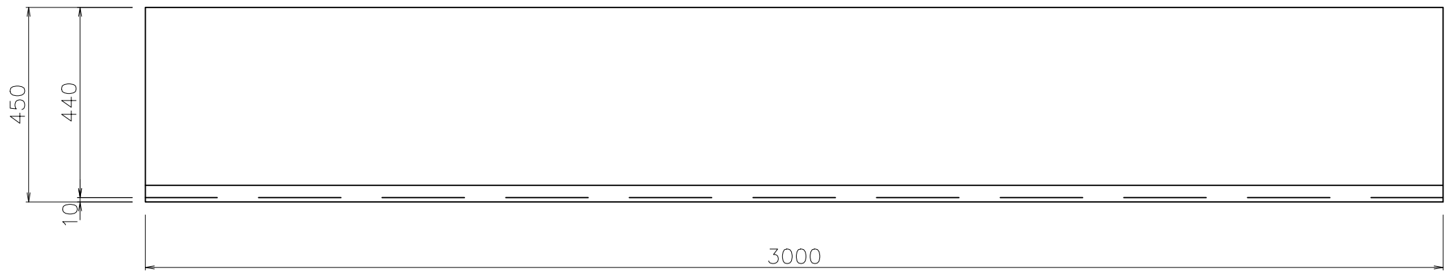
全 景 図 (S=1/6)
